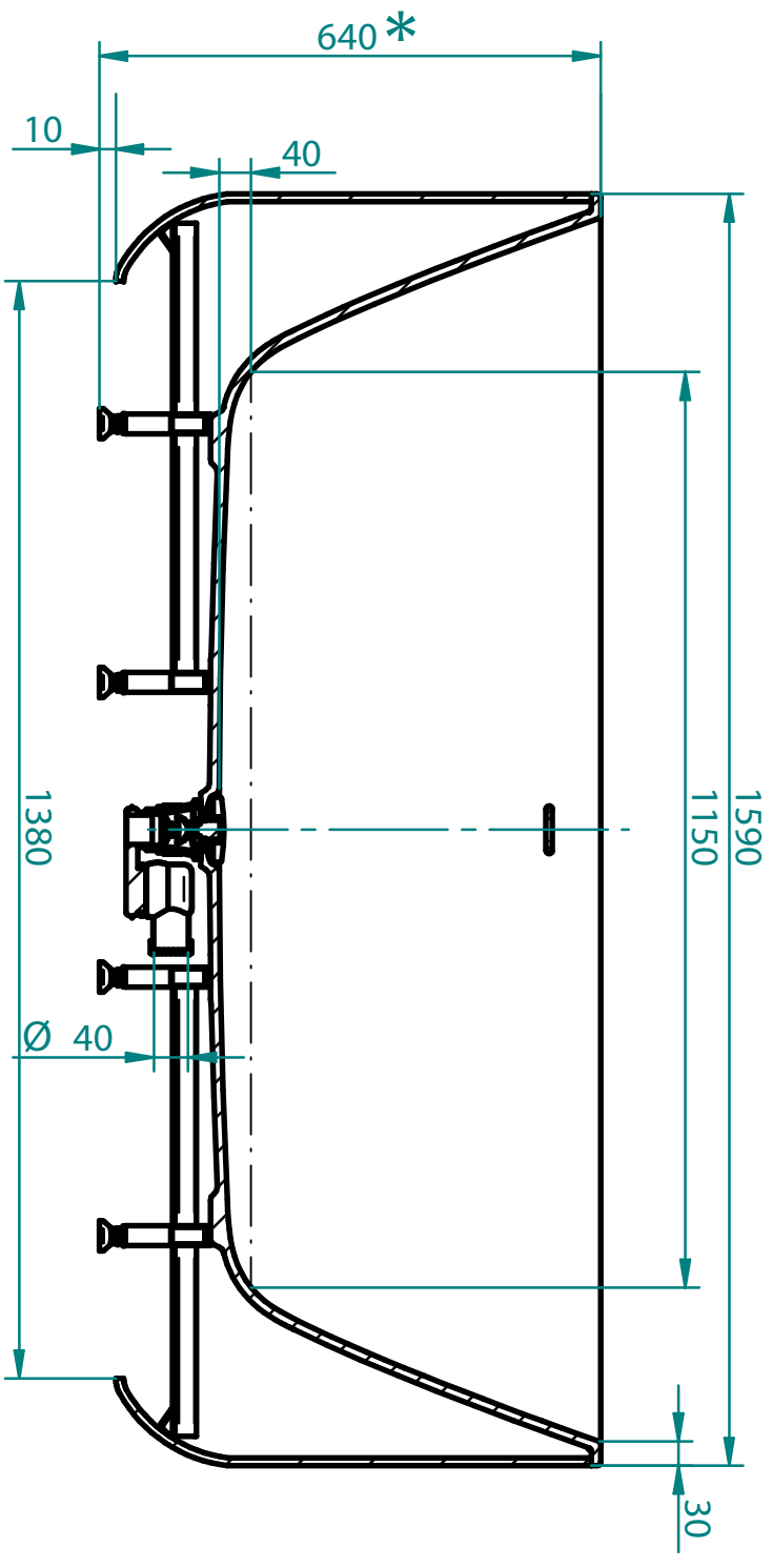
SECTION A-A
